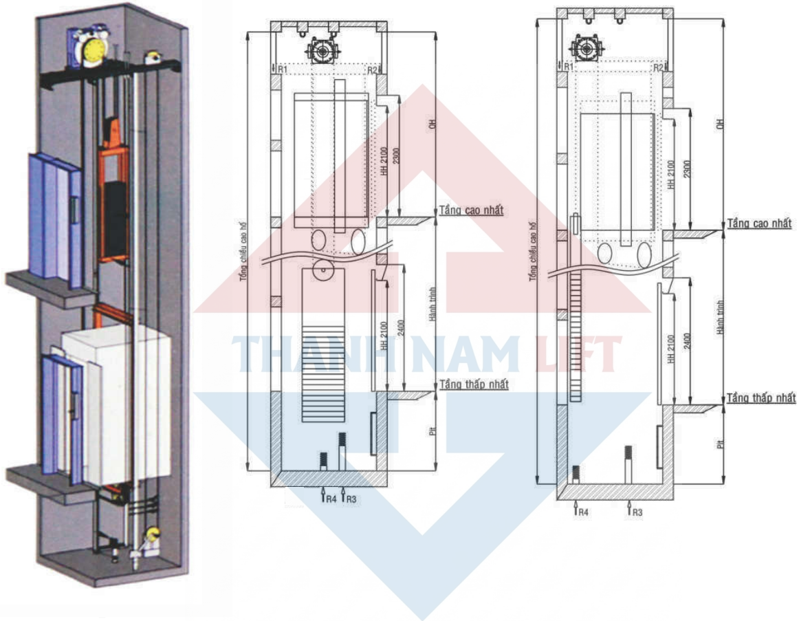
THANG TẢI KHÁCH ĐỐI TRỌNG PHÍA SAU
