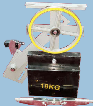
Bộ chống vượt tốc ( Governor )
