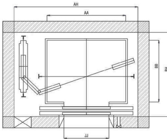
THANG TẢI KHÁCH ĐỐI TRỌNG BÊN HÔNG
